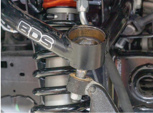
Fig. 14: Reattach the UCA.
